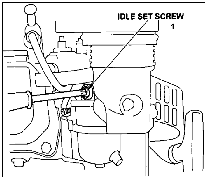
1 - винт регулировки холостого хода
