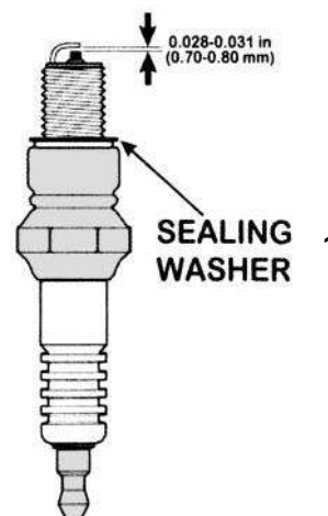
1 – уплотнительная шайба
