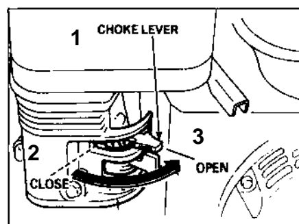
1 – рычаг воздушной заслонки 2 – закрыт 3 – открыт
